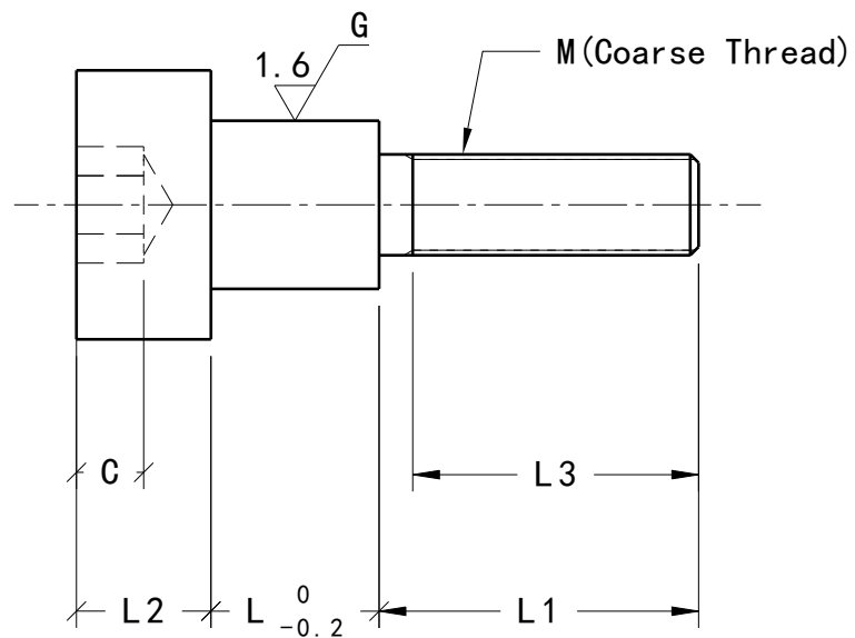
右視圖 縮放: 2:1
