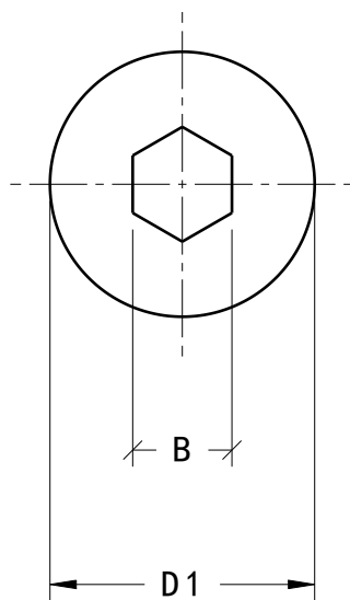
前視圖 縮放: 2:1
