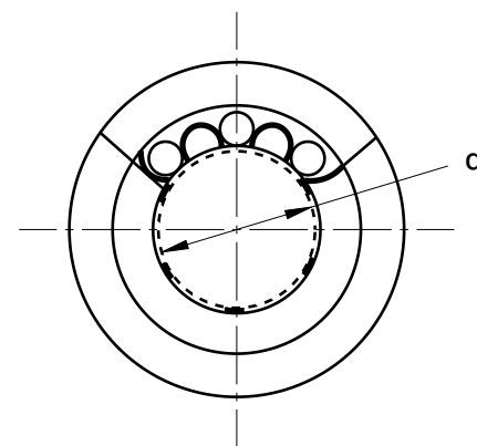
右視圖 縮放: 4:1
