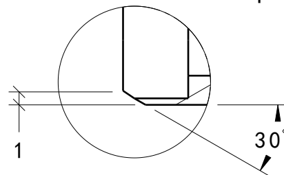
細部 B 縮放: 5:2
