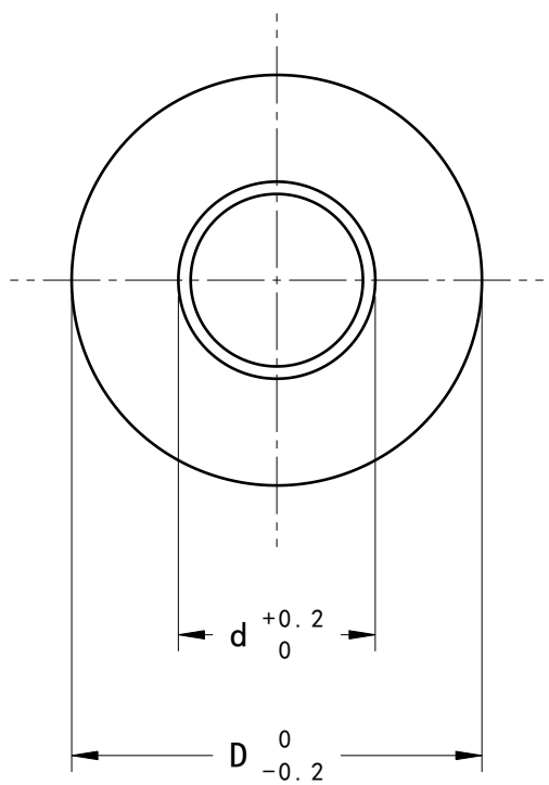
前視圖 縮放: 5:1
