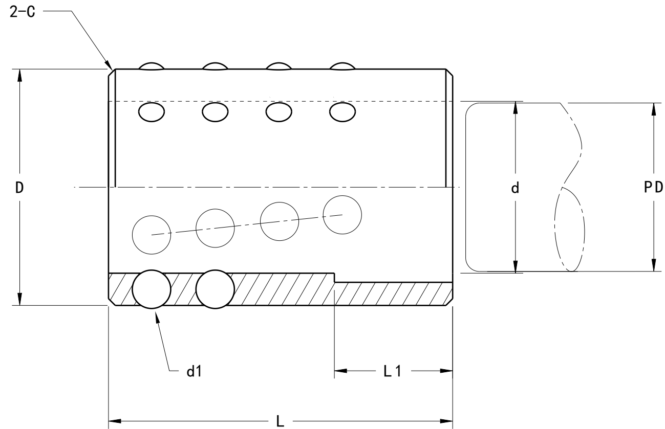
Section view A-A Scale: 7:4
