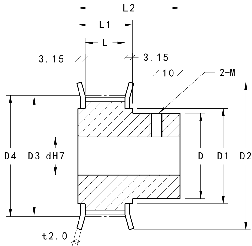
剖面視圖A-A 縮放: 1:1
