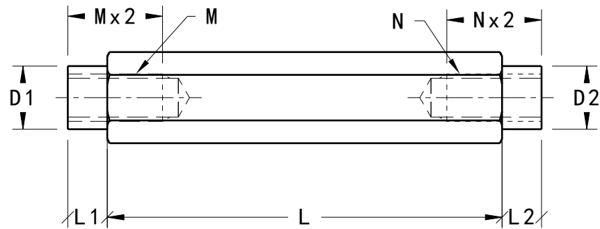
前視圖 縮放: 3:2
