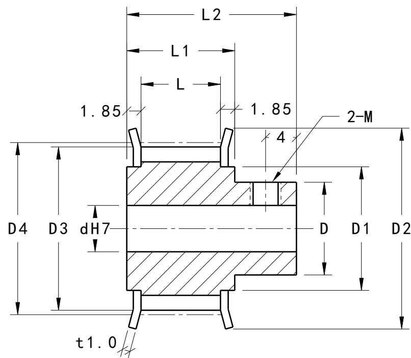
剖面視圖A-A 縮放: 2:1
