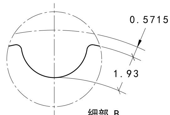
細部 B 縮放: 8:1
