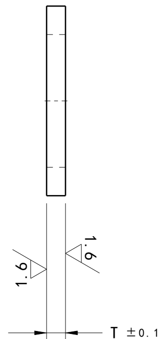
右視圖 縮放: 10:1
