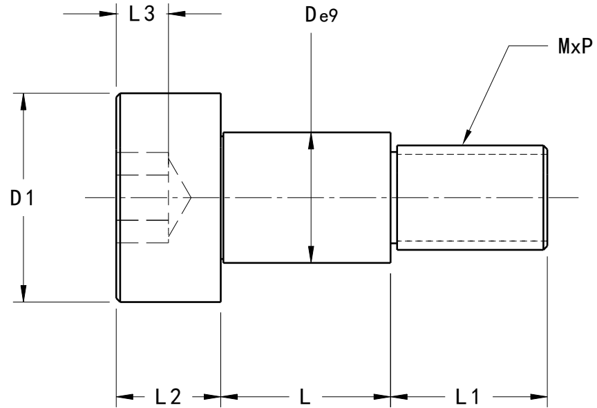
右視圖 縮放: 5:2
